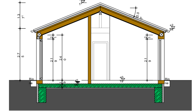
SCHNITT A-A Satteldach
