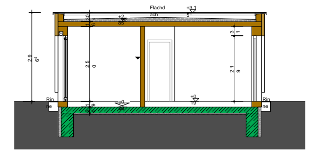
SCHNITT A-A Flachdach-Holzschalung
